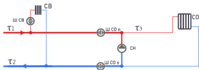
Рисунок 4 – Схема подключения потребителей к двухтрубной тепловой сети (при наличии внутренней системы отопления), СО – система отопления, СН – насос системы отопления, СВ – система вентиляции
