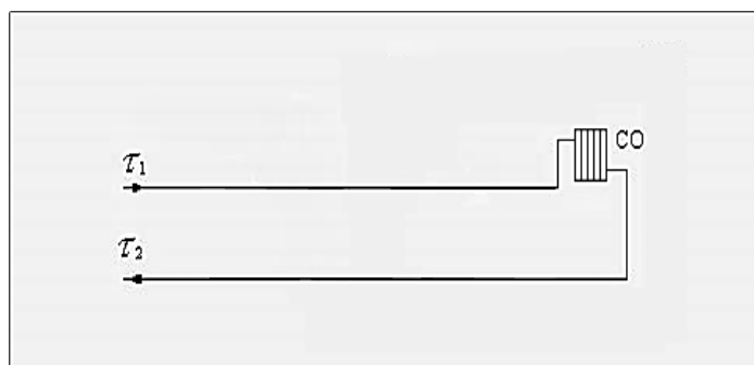
Рисунок 2 - Схема подключения потребителей к двухтрубной тепловой сети (при наличии внутренней системы отопления), зависимое присоединение, без смешения
